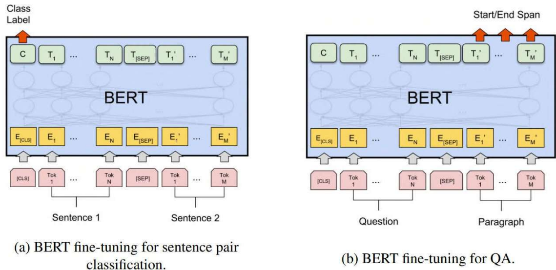
Fig 2.3 BERT finetuning
